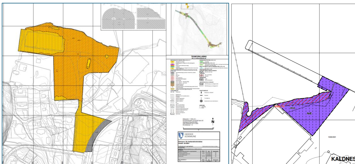
Figur 11 - Utsnitt fra plankart for ny fastlandsforbindelse fra Færder. Til venstre: Arealer regulert til midlertidig bygge- og anleggsområde i Færder kommune. Til høyre: Arealer regulert til næringsbebyggelse og bestemmelsesområde for midlertidig bygge- og anleggsområde i Tønsberg.
