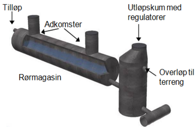
Figur 2; Prinsippskisse av rørmagasin
