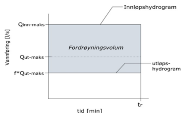
Figur 10. Regnevelopmetoden med antatt konstant innløp og utløp. Regnvarighet, t_r .
