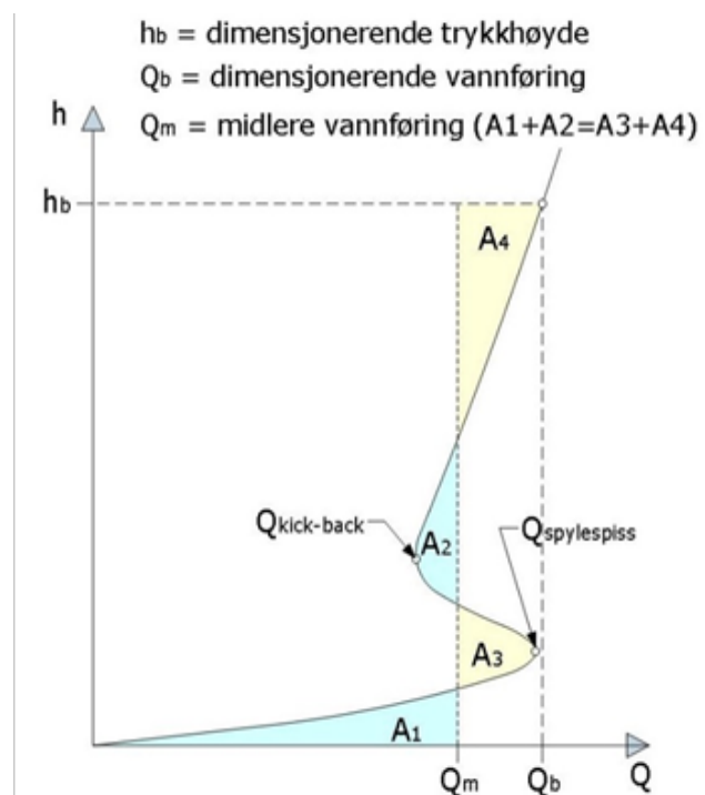
Figur 4. Viktige parametere: Q_b , h_b , Q_m .
