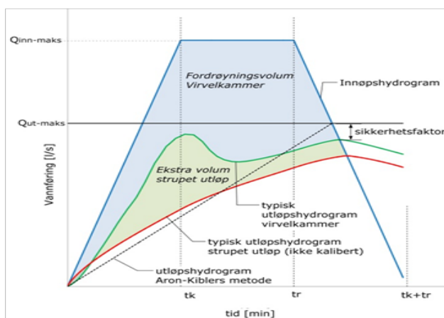
Figur 11. Regnevelopmetoden med varierende utløp for et typisk virvelkammer (Aron-Kibler innløpshydrogram, konsentrasjonstid t_k ).
