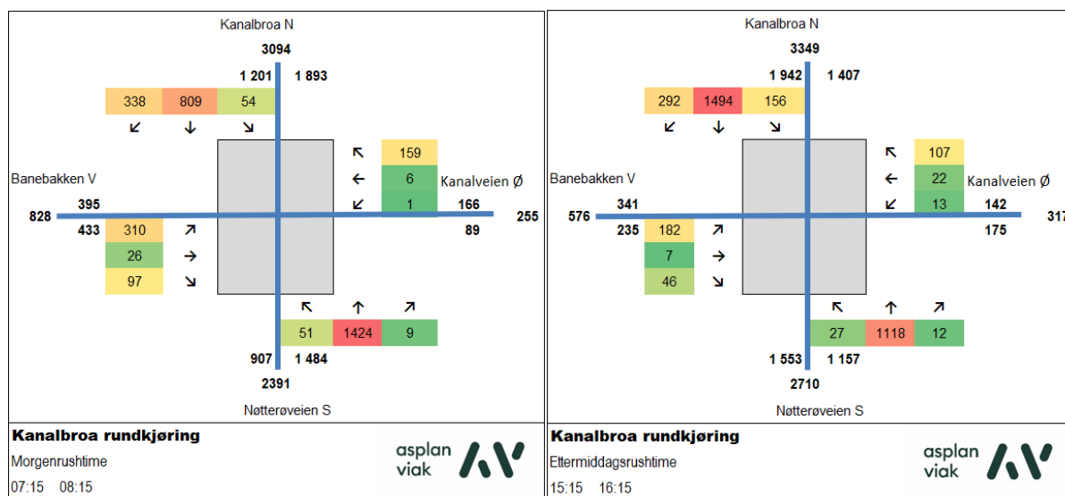
Figur 2-13 Oversikt av rushtimetrafikk for både morgen- og ettermiddagsperiodene. Tallene viser timetrafikk per svingebevegelse og summert per veiarm inn og ut av rundkjøringen
