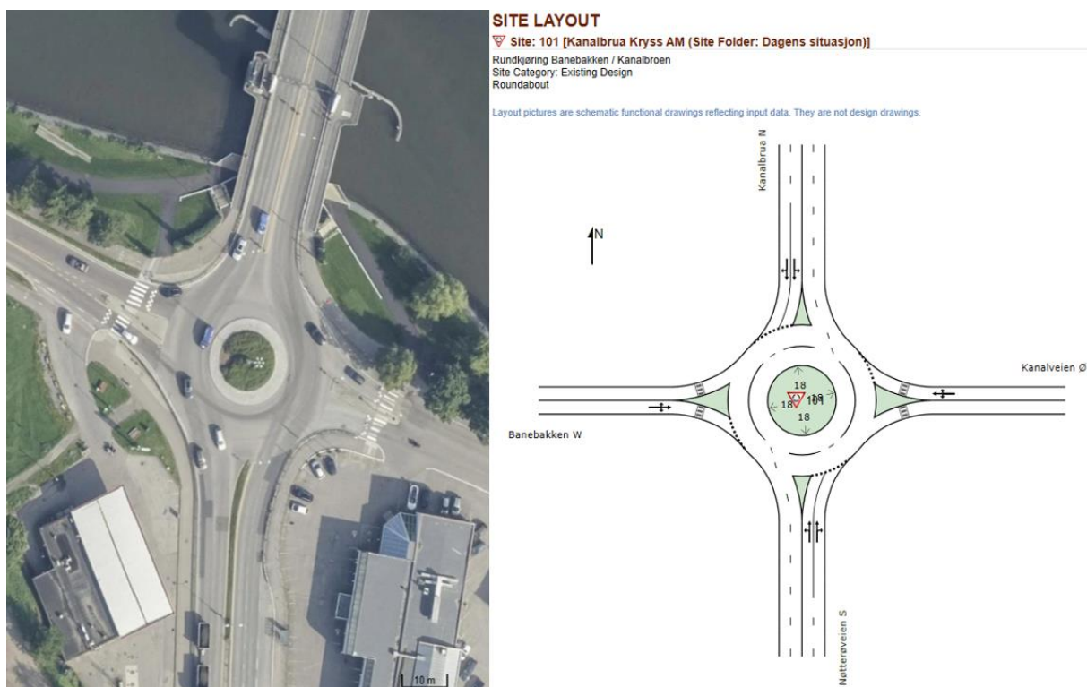
Figur 5-7 Dagens kryssutforming i Kanalbrua rundkjøring
