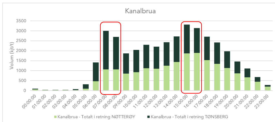
Figur 2-9 Timetrafikkfordeling Kanalbrua kontinuerlig tellepunkt. Oktober 15. 2024
