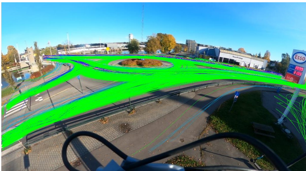
Figur 2-11 Kjøretøybane-analyse i Goodvision for ettermiddagsperioden
