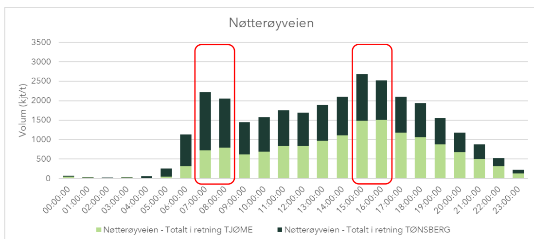
Figur 2-10 Timetrafikkfordeling Nøtterøyeveien kontinuerlig tellepunkt. Oktober 15. 2024
