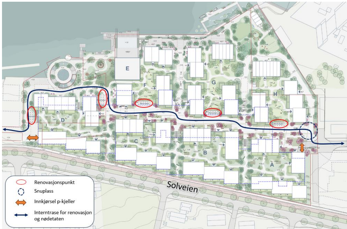
Figur 7-2 Internløsninger for renovasjon, nødetaten og kjellerparkering
